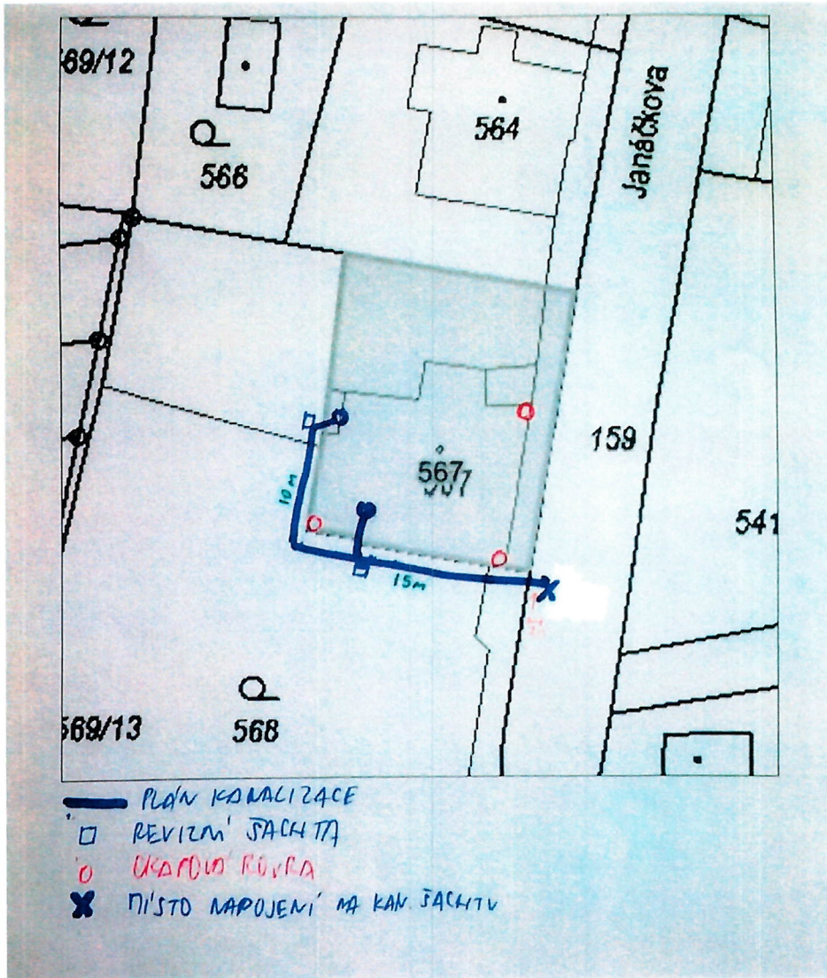
Příloha č. 5 – Situační plán se zakreslením zamýšleného napojení kanalizační přípojky
