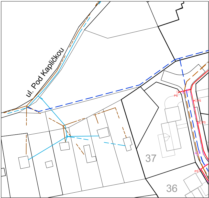
VÝŘEZ - NAPOJENÍ V ULICI POD KAPLIČKOU - 1:1000
